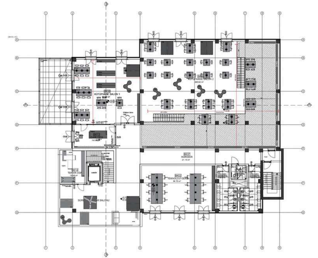
Asma Kat Planı (+8.00 Kotu) h:300 cm 1/50
