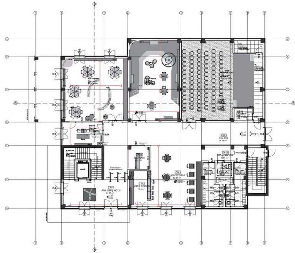
Zemin Kat Planı (±0.00 Kotu) h:500 cm İnş. Alanı : 661.59 m 2 1/50
