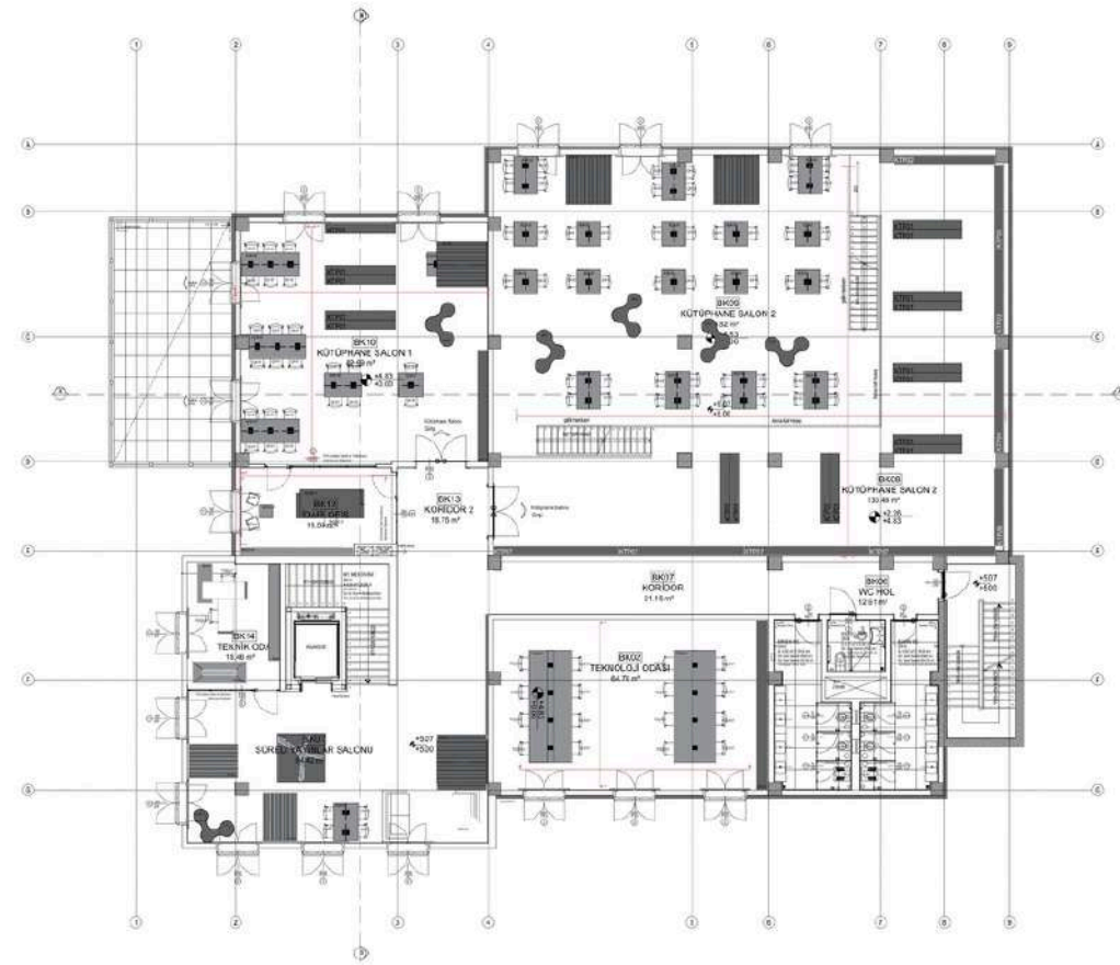
1. Kat Planı (+5.00 Kotu) h:600 cm İnş. Alanı :747.84 m 2 1/50
